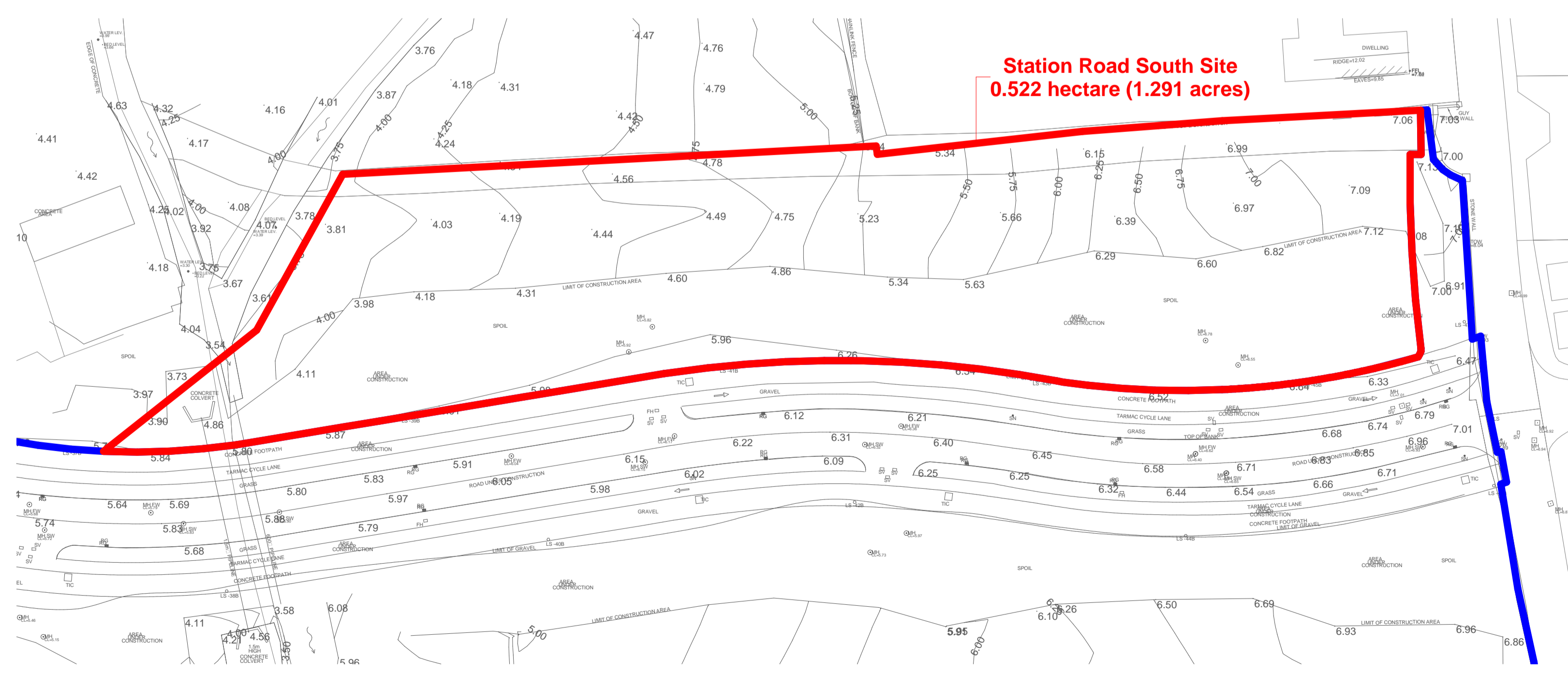
2 Existing Site Survey 08 1 : 500
